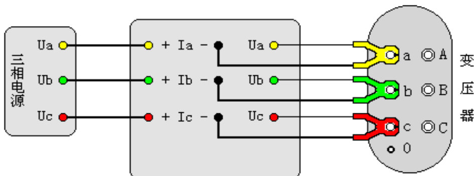
图十九 三相电源测量变压器空载损耗
