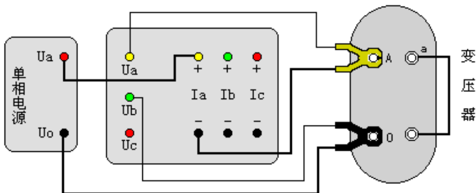
图二十 单相变压器短路损耗测量
