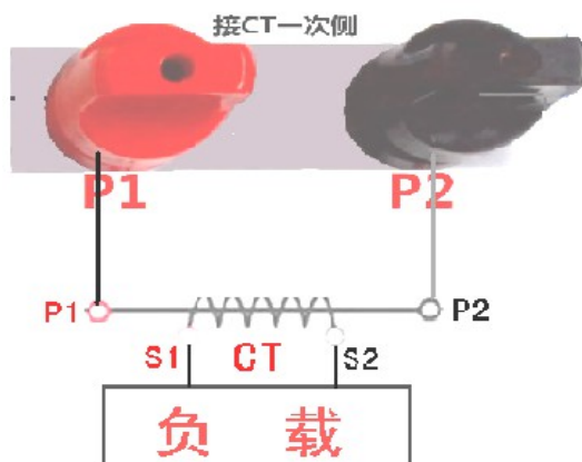
图 14、CT 一次通流接线图
