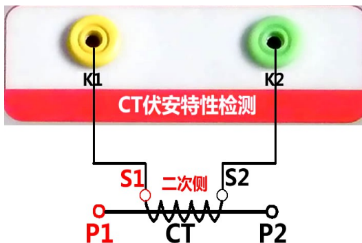
图 4，CT 励磁特性接线图
