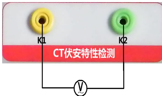
图 21，电压校准接线图
